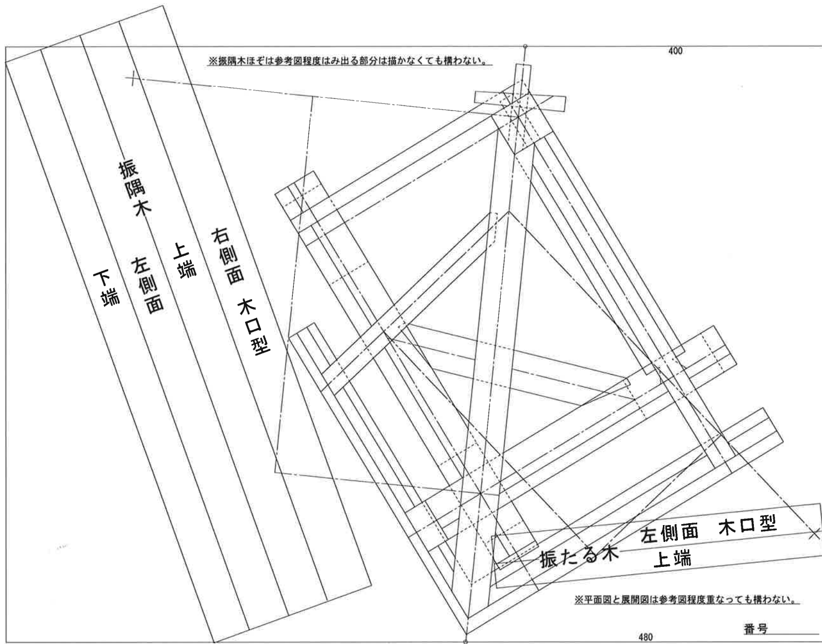
現寸図配置参考図
