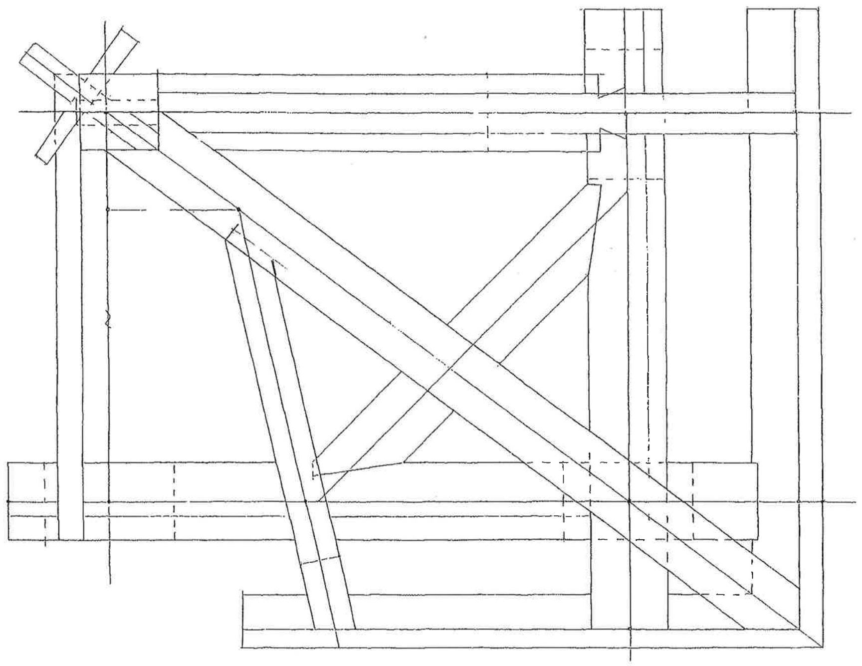
振隅木平面図
